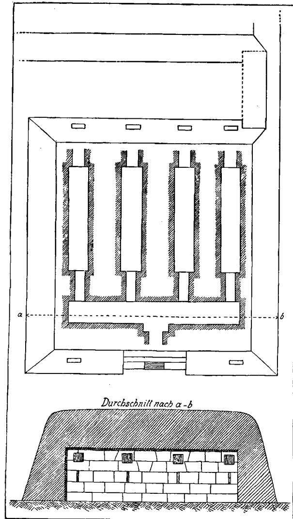
Abb. 63. Statuenhaus des Btftb, Plan und Schnitt.
