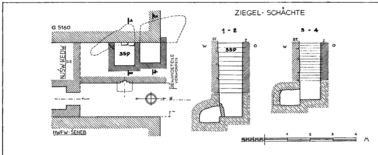
Abb. 52. Mastaba S 359, Grundriß und Schnitte.
