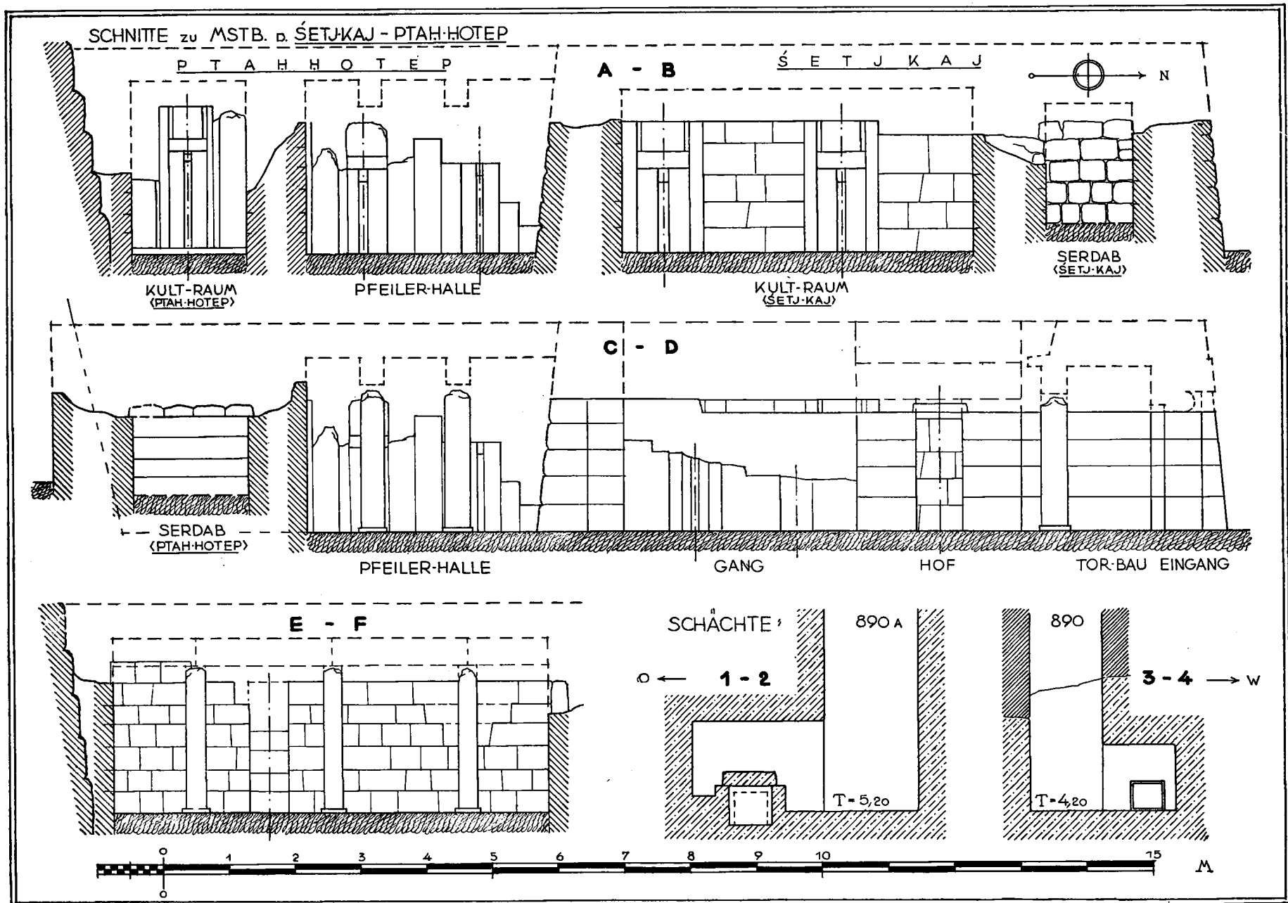
Abb. 84. Die Mastaba des Šetjka und Ptahhotep, Schnitte.
