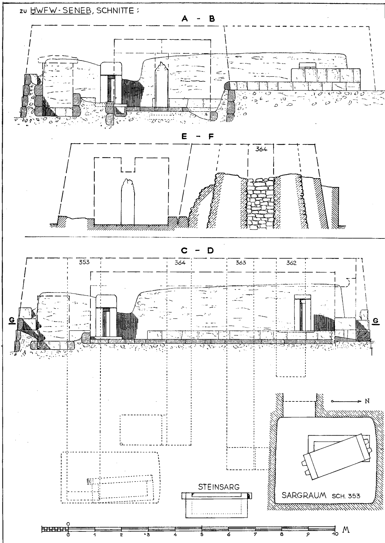
Abb. 44. Die Mastaba des Hefwesh I , Schnitte.
