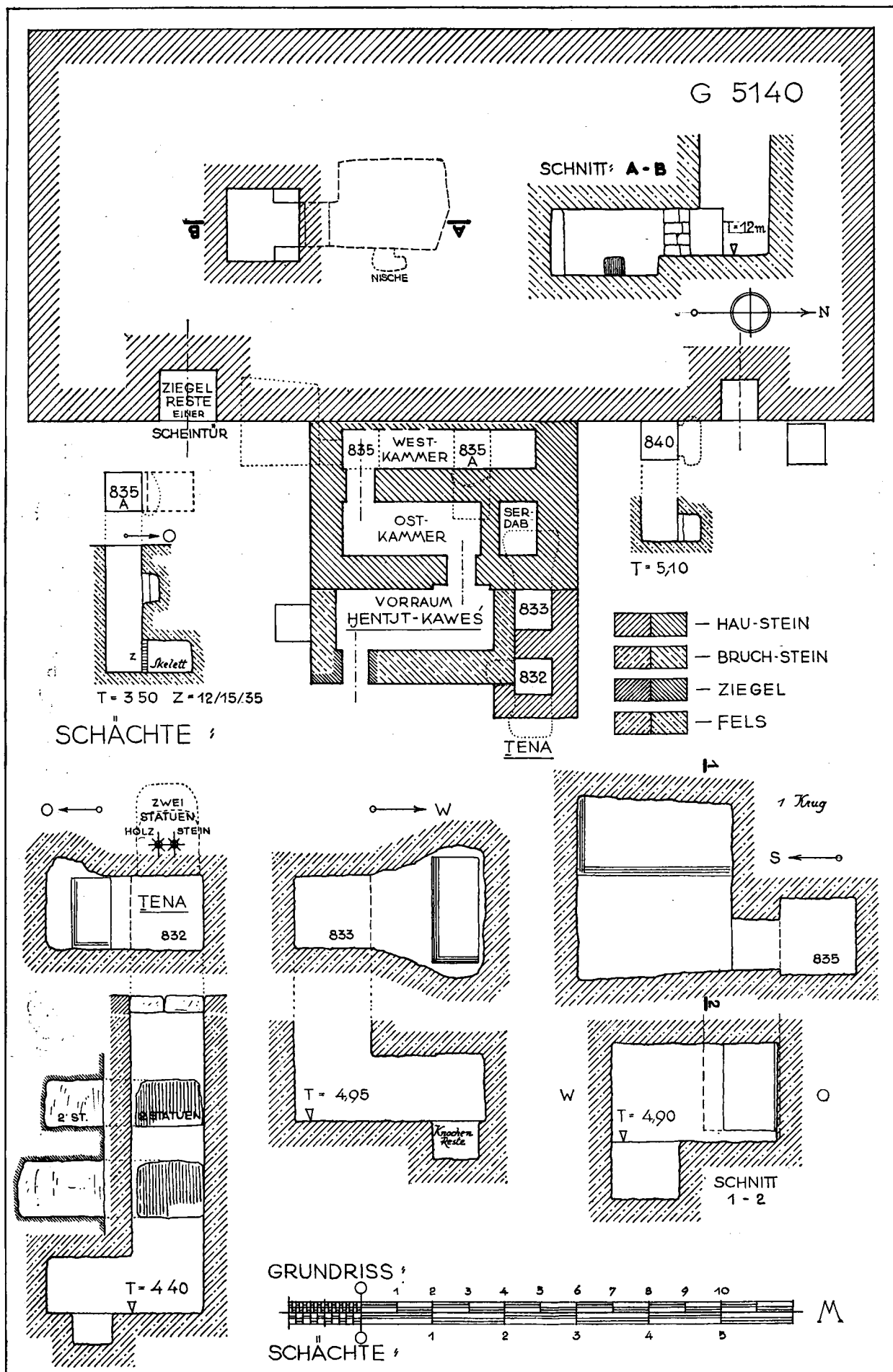
Abb. 28. G 5140 und die Maßstäbe der Hutkwa , Grundriß und Schnitte.
