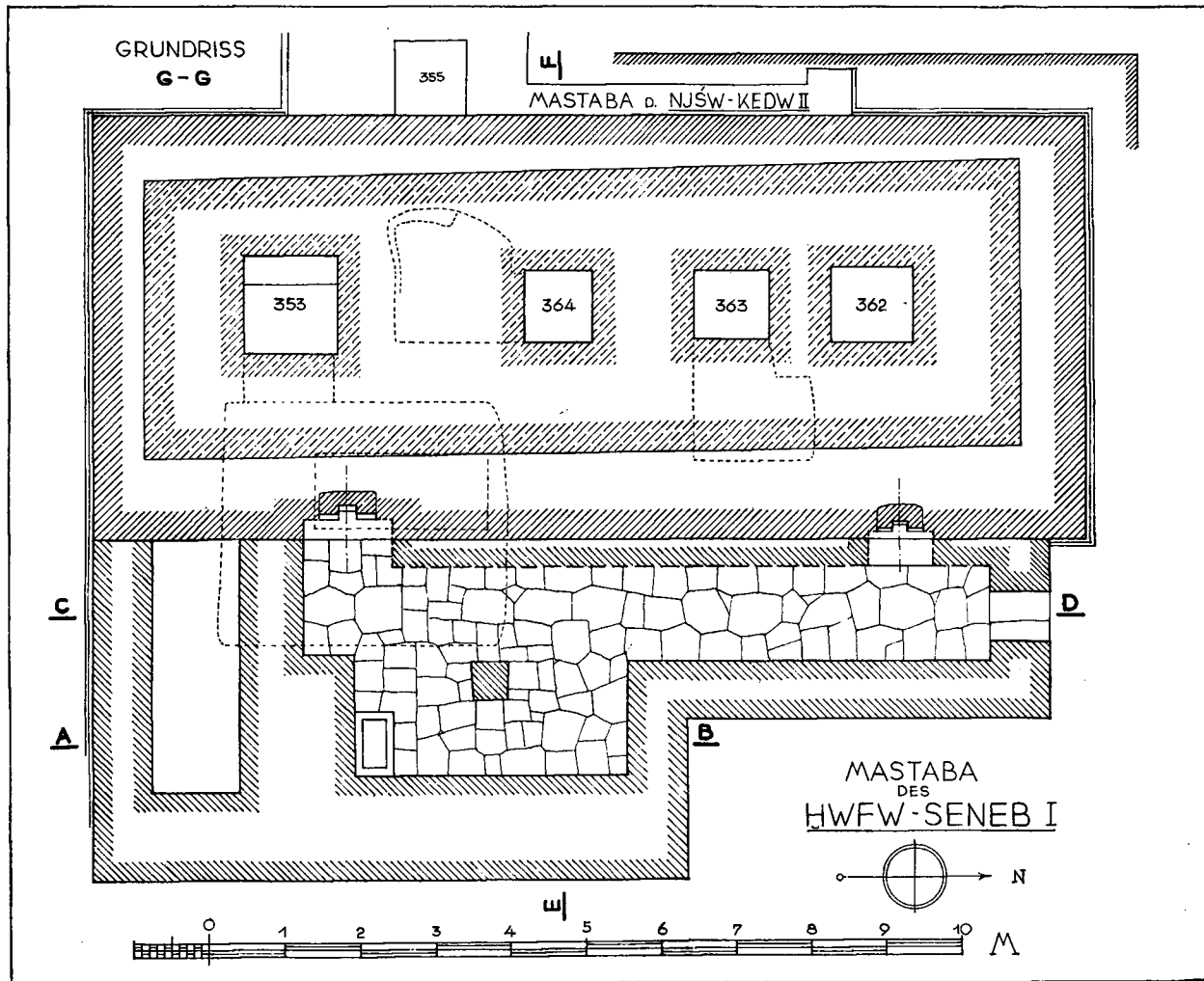
Abb. 43. Die Mastaba des Hufwšnb I , Grundriß.
