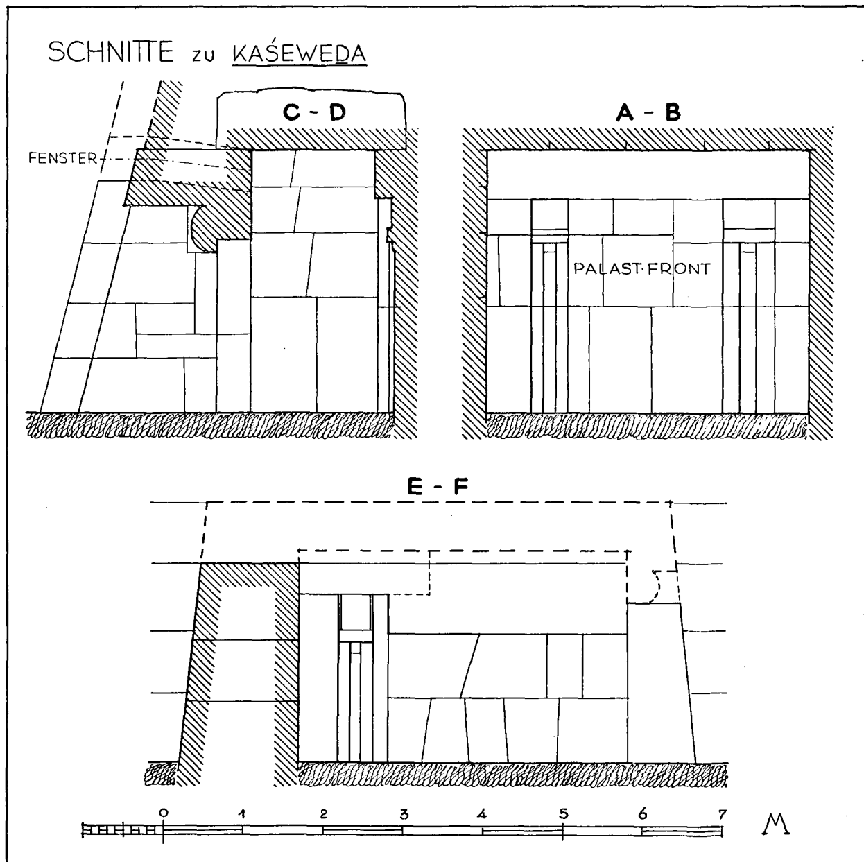
Abb. 68. Die Mastaba des Kheswesi , Schnitte.
