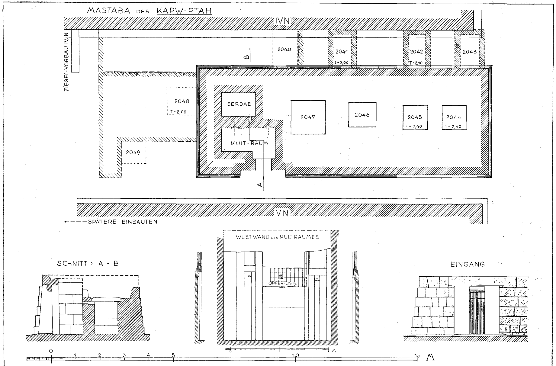
Abb. 87. Die Mastaba des Kpw-ptah , Grundriß und Schnitte.
