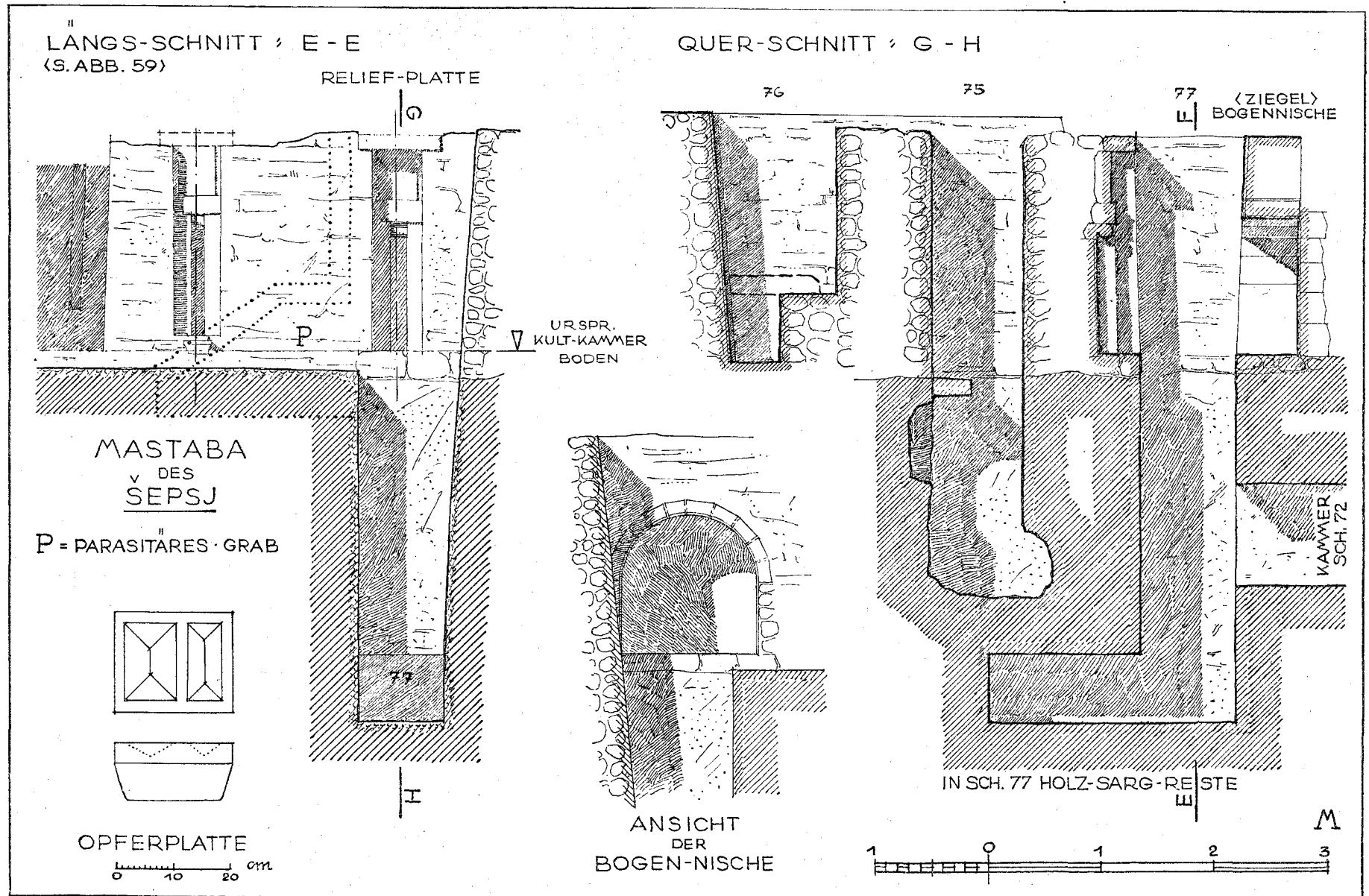
Abb. 61. Die Mastaba des Špsj, Schmitte.
