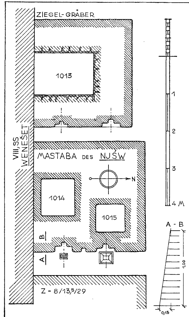
Abb. 99. Die Mastaba des Njśw und Mastaba S 1013, Grundrisse.
