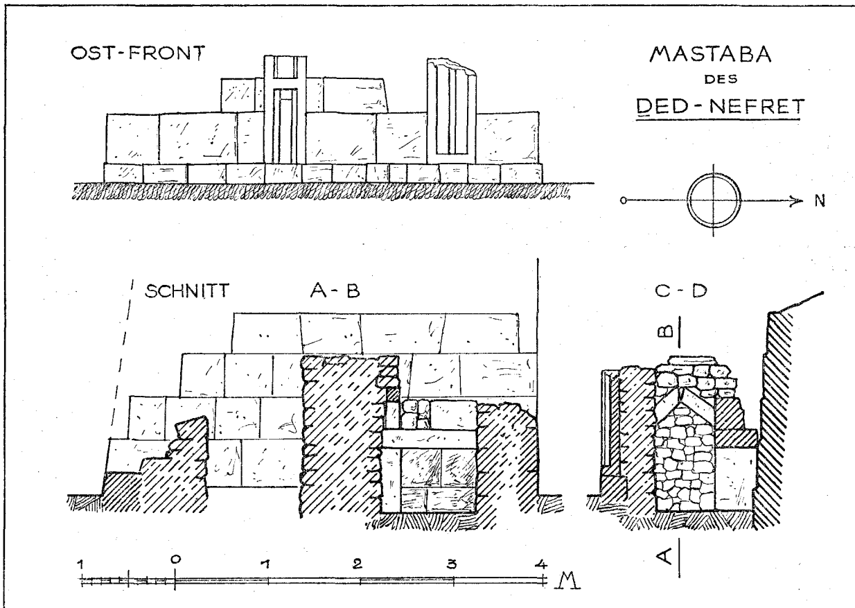
Abb. 48. Die Mastaba des Dendefret , Ansicht und Schnitte.
