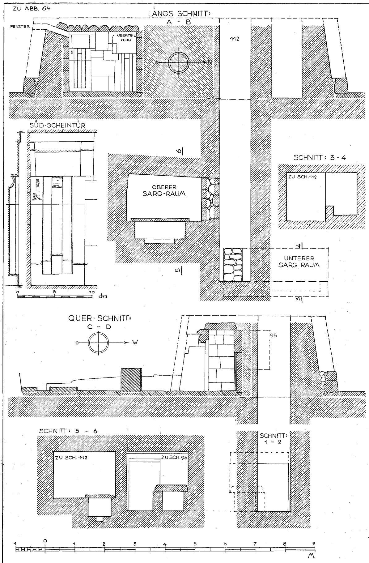
Abb. 65. Mastaba S 95/112, Schnitte.
