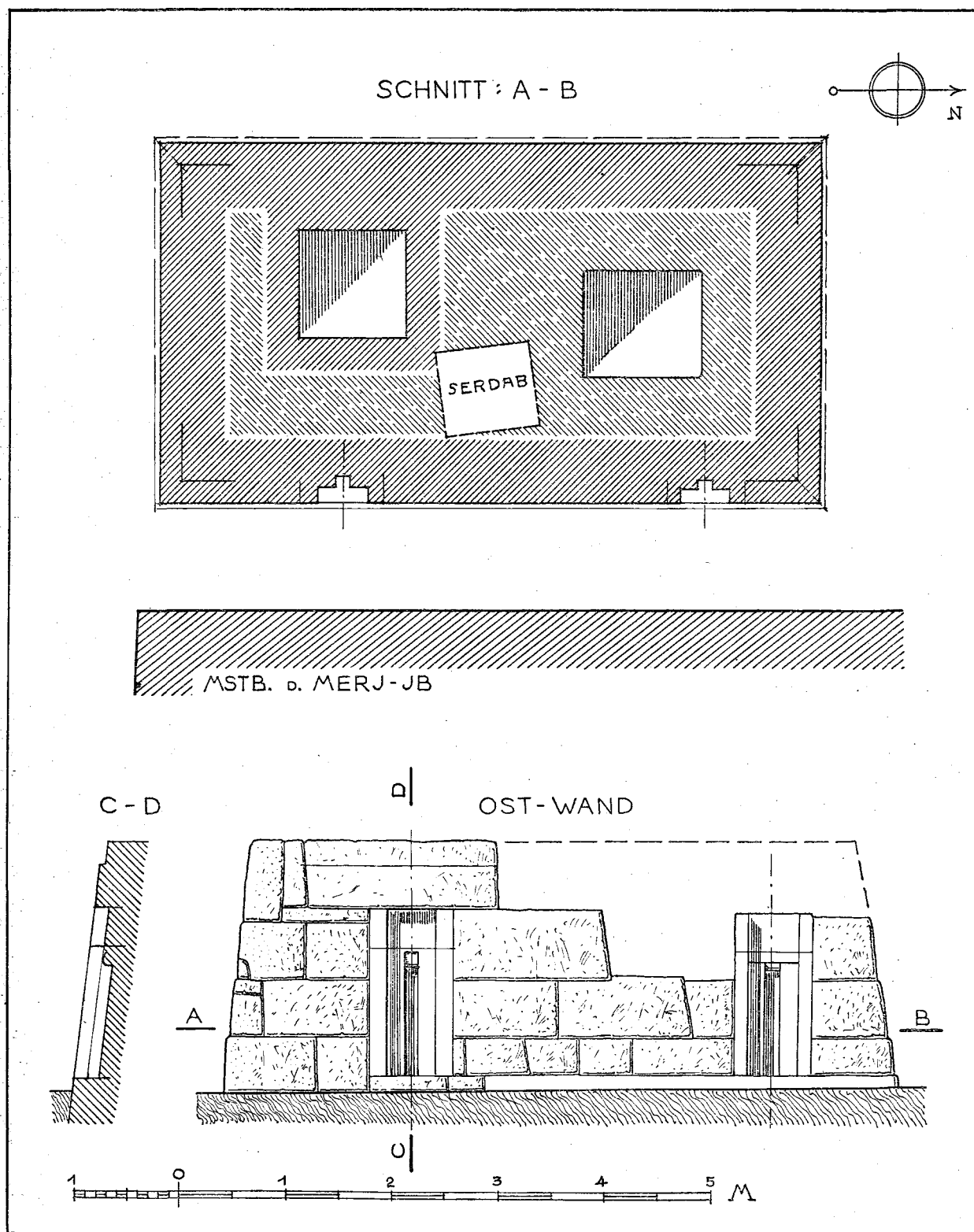
Abb. 77. Maṣṭaba westlich von Mrjib .
