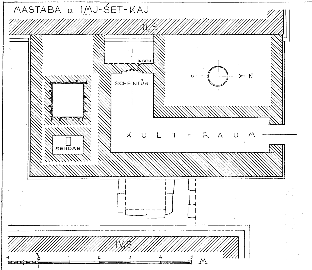
Abb. 80. Die Mastaba des 'Imjstktj, Grundriß.
