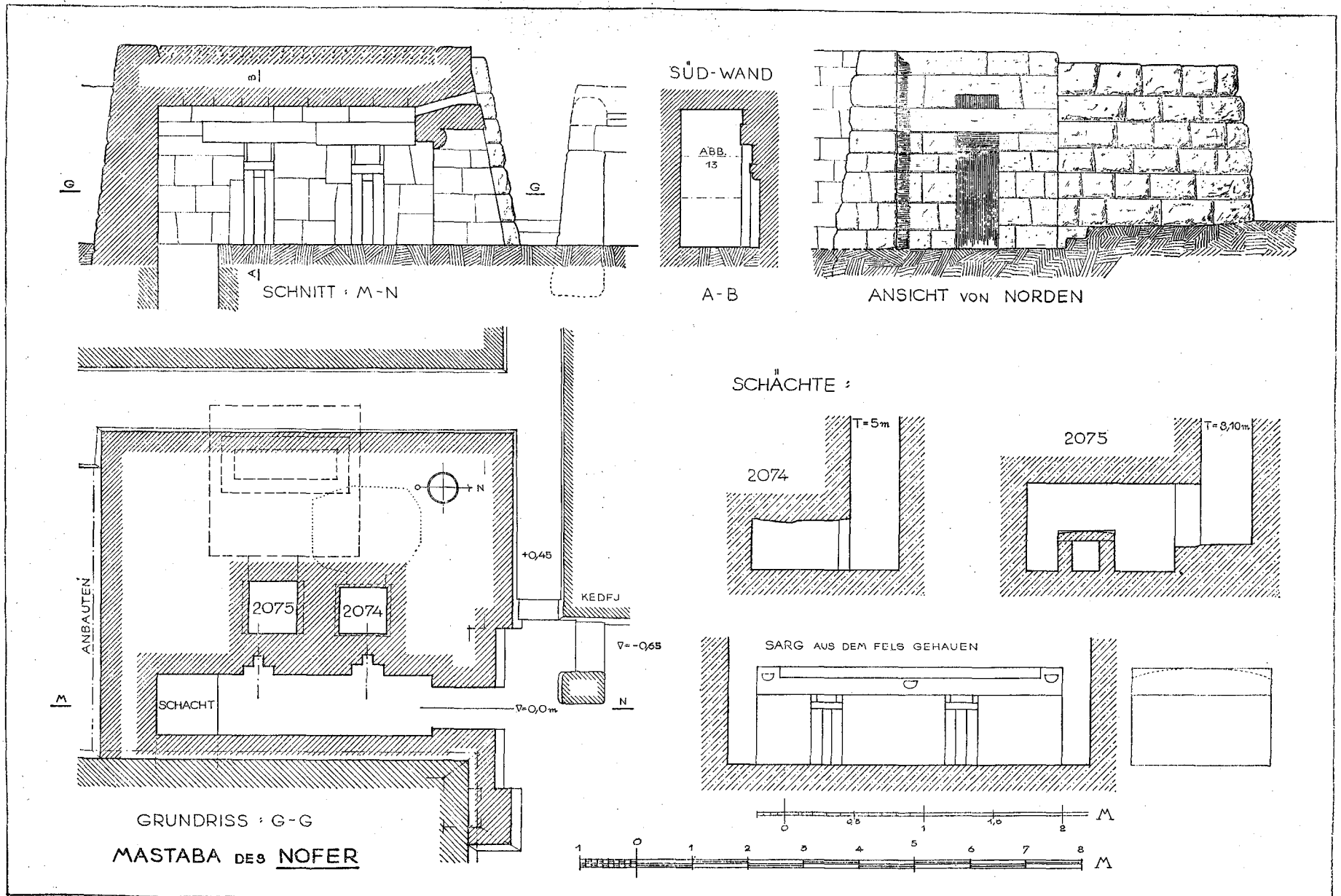
Abb. 3. Die Mastaba des Nfr , Grundriß und Schnitte.
