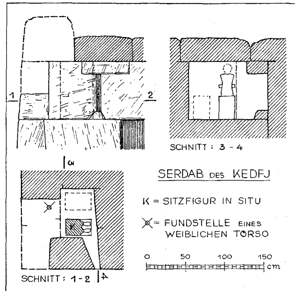
Abb. 24. Die Mastaba des Kdfj , Serdab.
