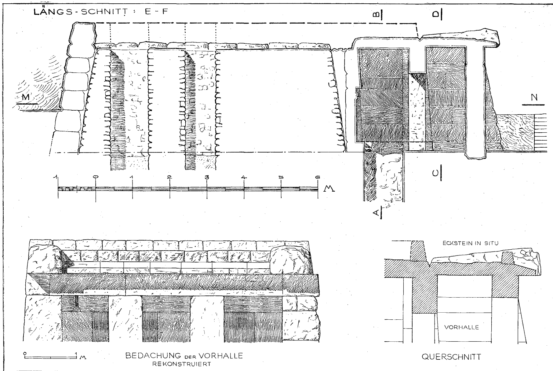
Abb. 22. Die Mastaba des Kdfjy, oben Längsschnitt, unten Bedachung.
